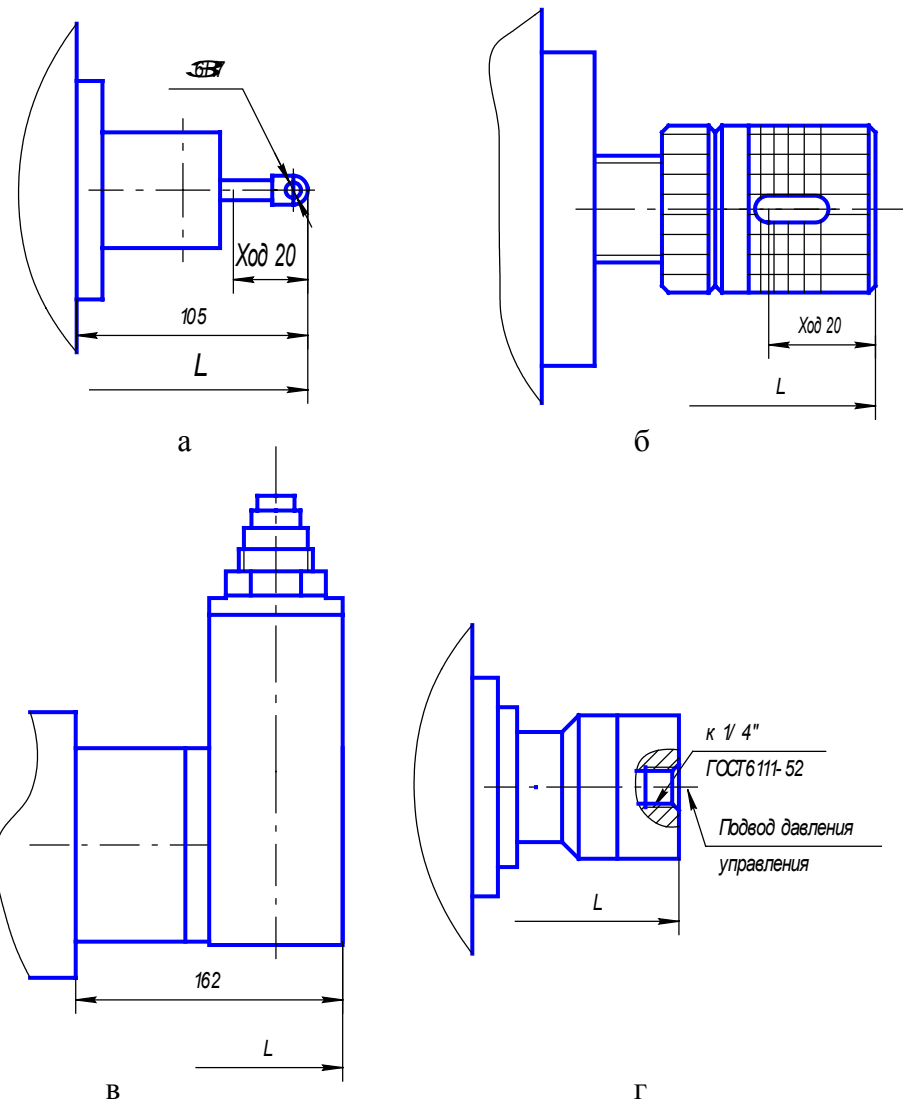
Рисунок 3 – Механизмы изменения подачи а – следящего управления 50НРР...С; б – ручного управления 50НРР...Р; в – регулятор мощности 50НРР...Д1; г – гидравлического управления 50НРР...Г
