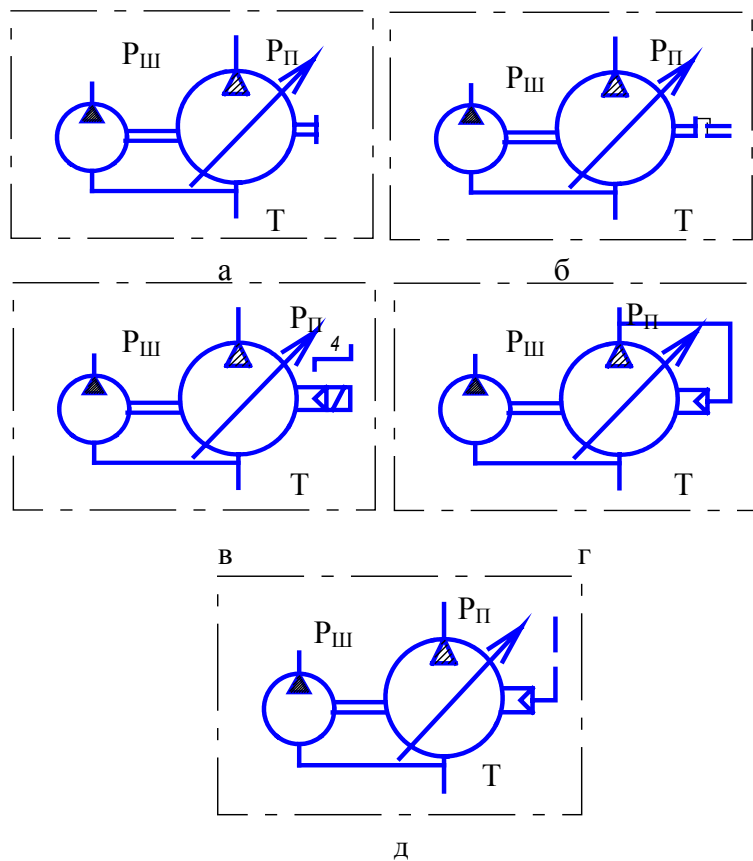
а – 50НРР...Р; б – 50НРР ...С; в – 50НРР ...М; г – 50НРР ...Д1; д - 50НРР ...С
