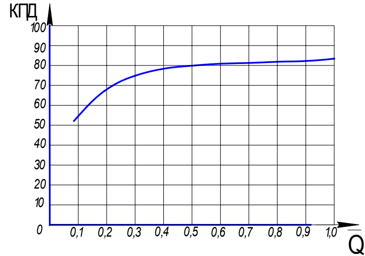
Рисунок 6 – Зависимость КПД поршневого насоса от подачи при номинальном давлении
