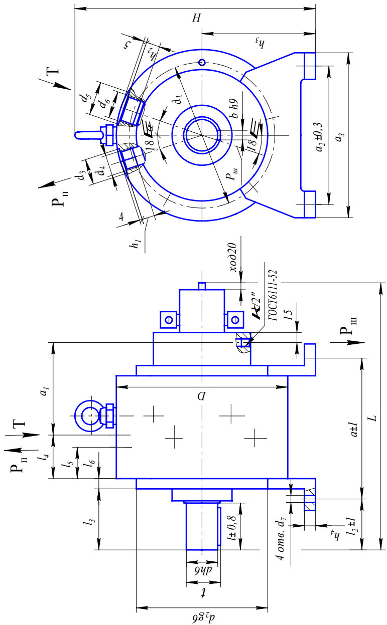
Рисунок 2 – Габаритные и присоединительные размеры насосов 50НРР с электромагнитным механизмом изменения подачи
